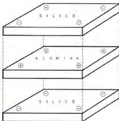
Figura 10. Elemento de arcilla Montmorillonita (esquema)
