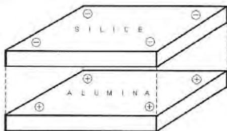
Figura 9. Elemento de arcilla Caolinita (esquema)
